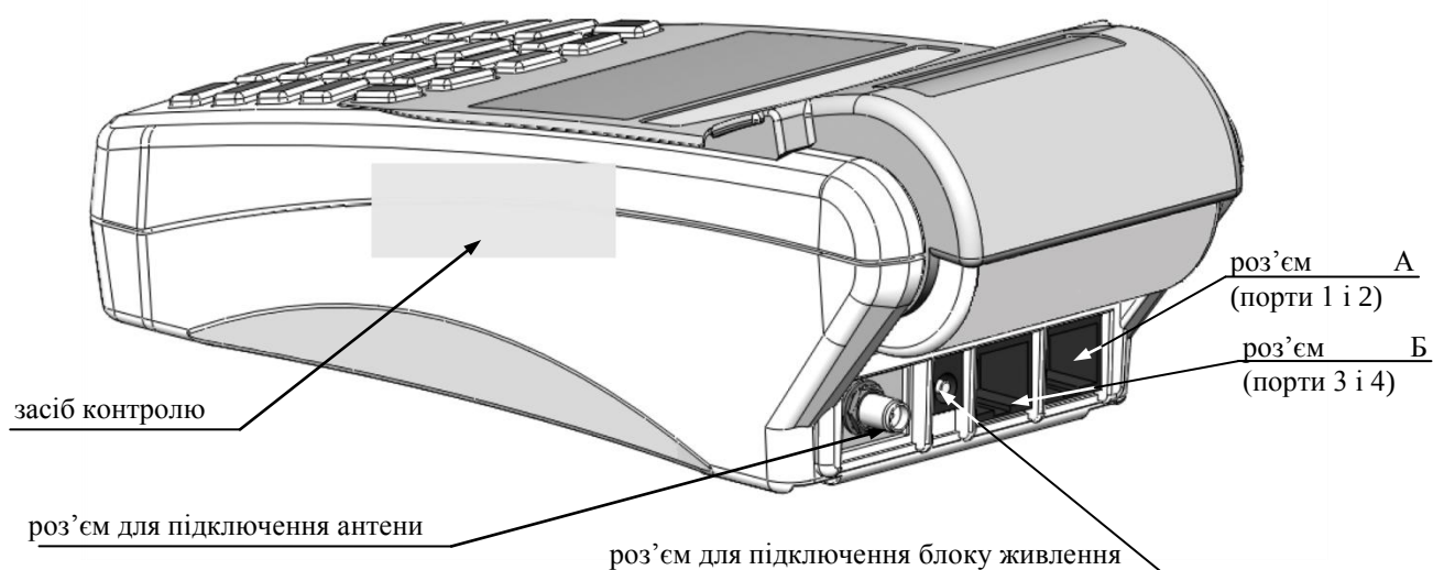
Рис. 2 Вид з боку
