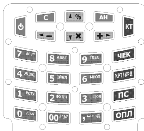
Рис. 4 Клавіатура ЕККА MINI-T 400ME з
