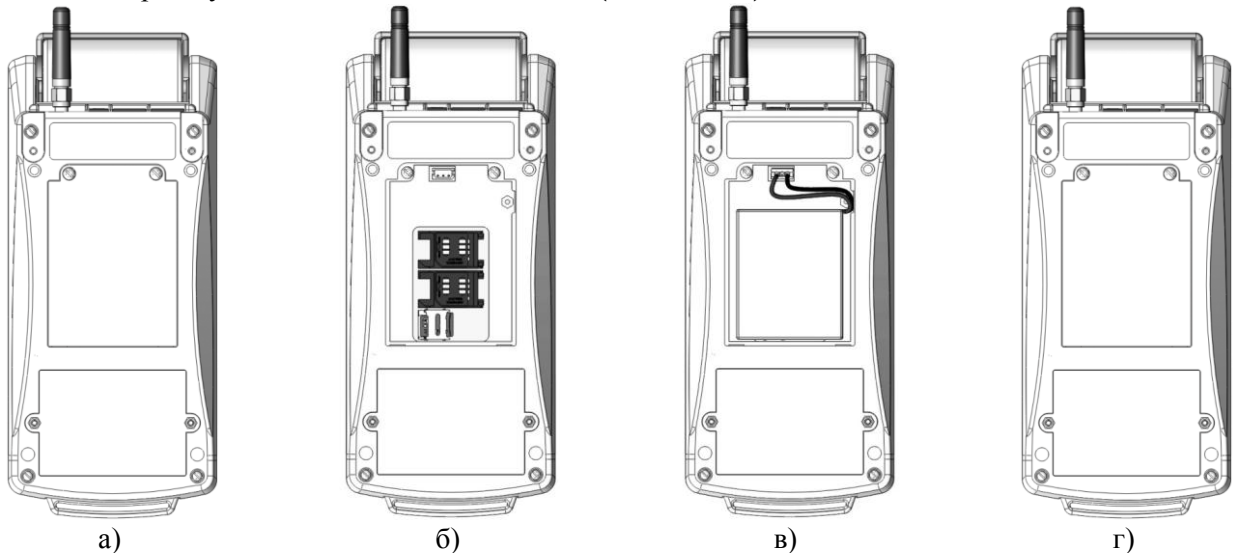
Рис. 7 Встановлення акумуляторної батареї в касовий апарат
